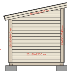
Обшивка. Вид слева
