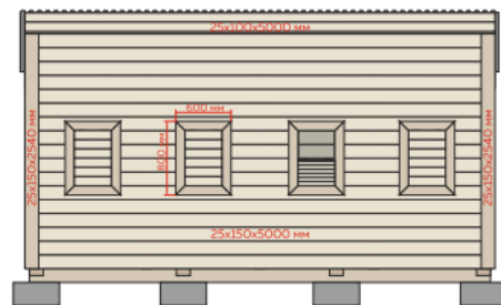
Обшивка. Вид спереди
