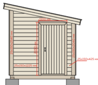
Обшивка. Вид справа
